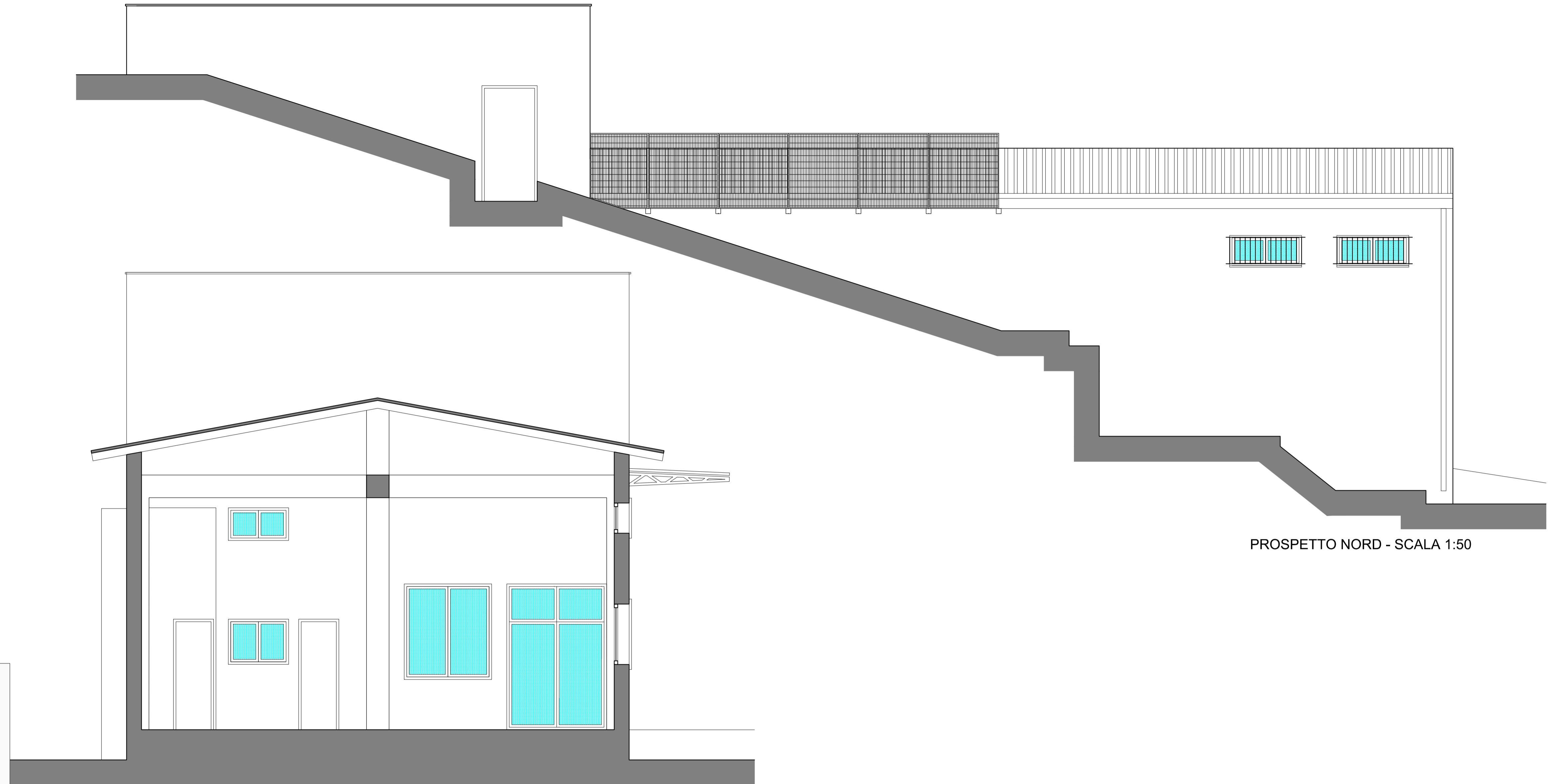
SEZIONE TRASVERSALE - SCALA 1:50
