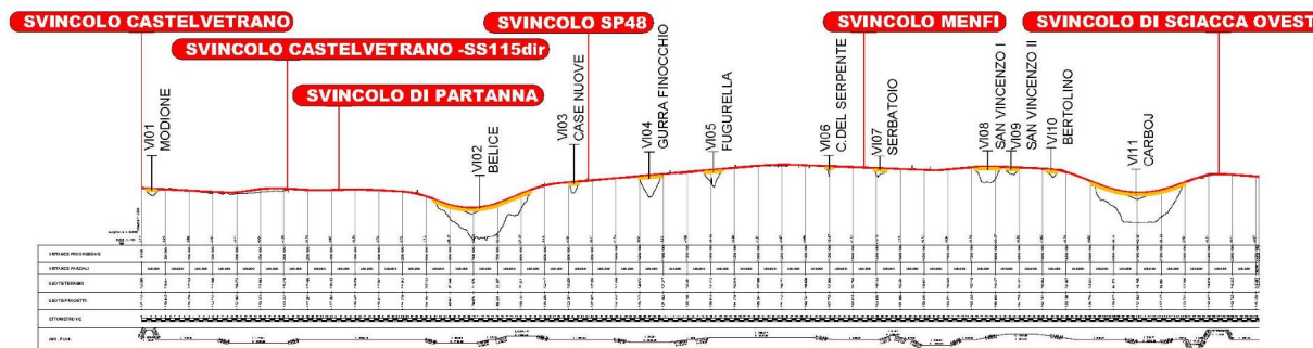
Figura 3-9 – Planimetria e profilo di progetto – Alternativa 2A
