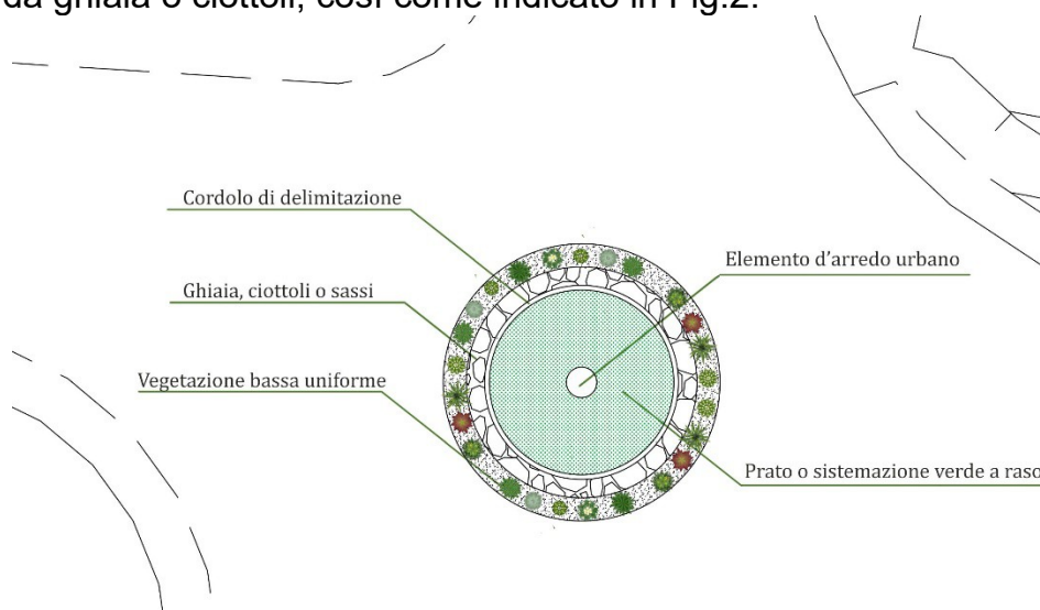
Fig.2 Schema tipo sistemazione rotonda a raso con allestimento misto ridotto e snello
