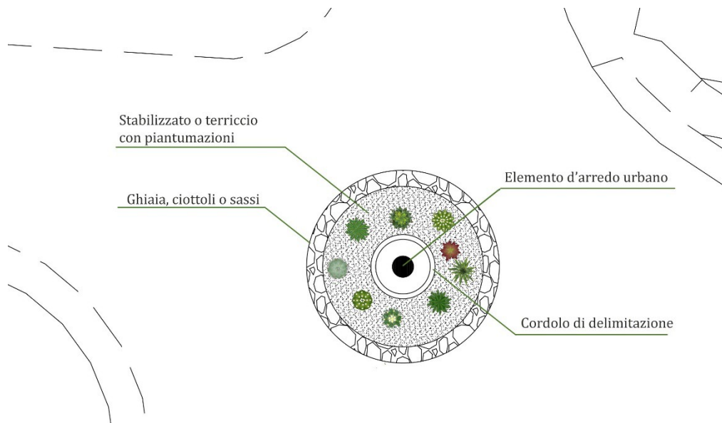
Fig.1 Schema tipo sistemazione rotonda a raso con allestimento snello
